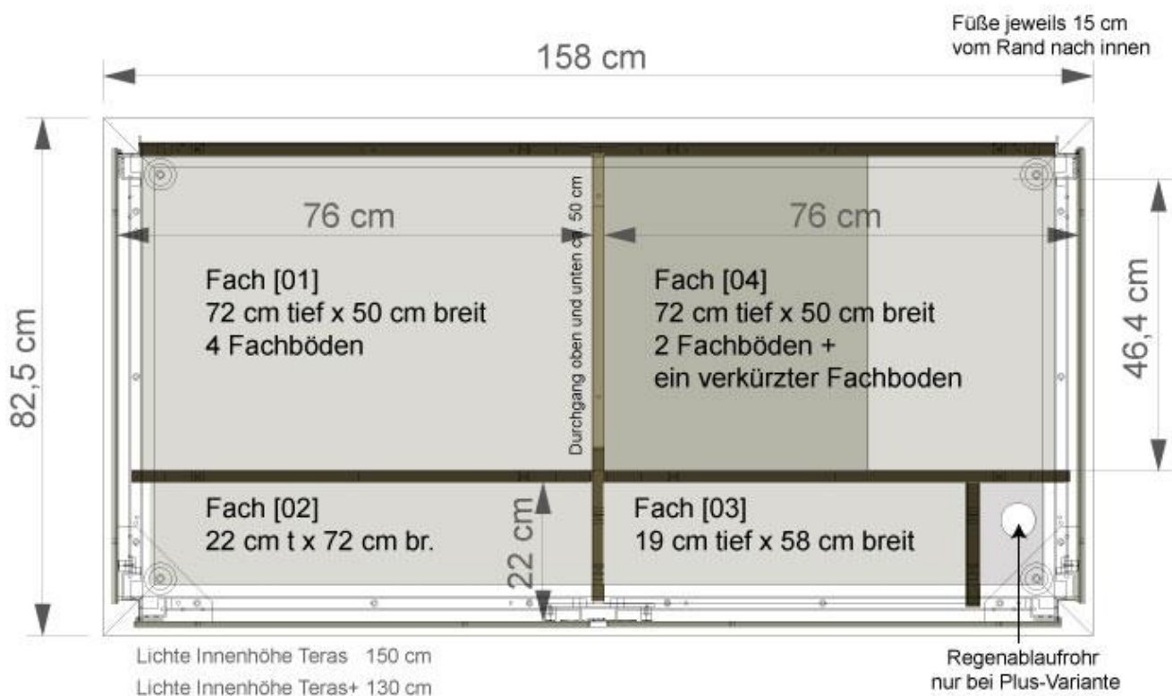
Grundriss Garten[Q]Teras in der Standardausführung mit Zugriff von drei Seiten
